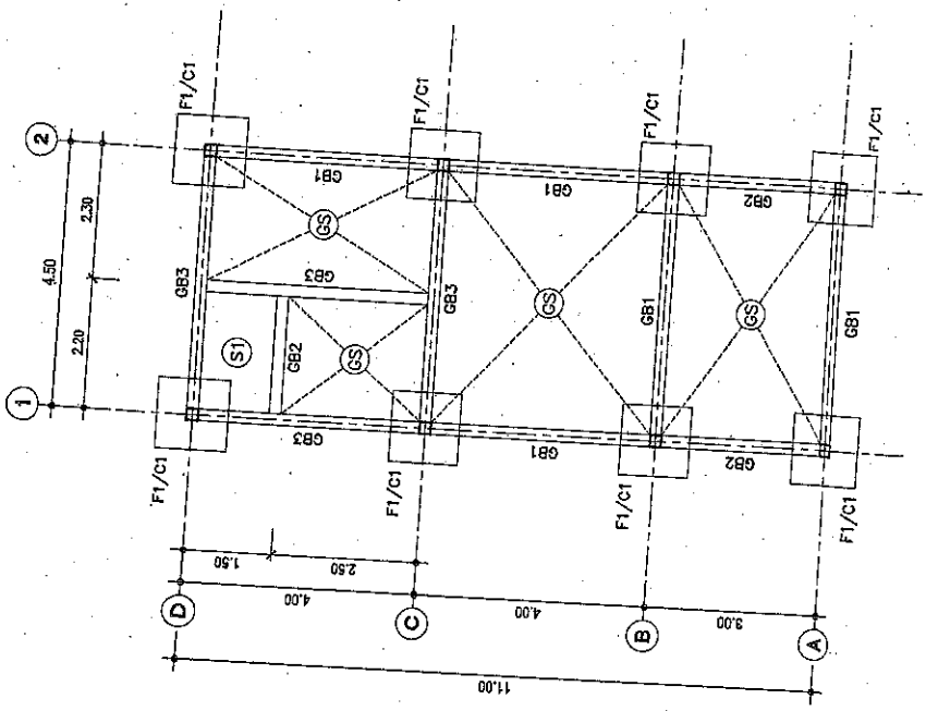
แปลนฐานราก, เสา, คาน, พื้น มาตราส่วน 1:100
