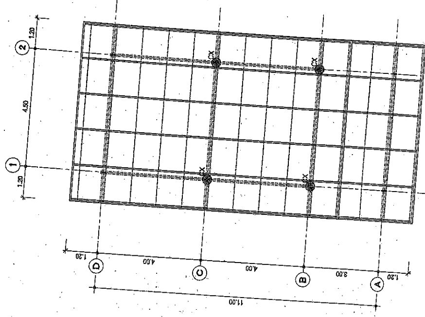
แปลนโครงหลังคา มาตราส่วน 1:100
